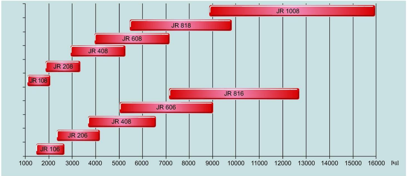
Konstruktionsgewicht bei Einsatz eines Richterreggers – Construction weight when using one exciter – Poids du châssis vibrant lors de l'utilisation d'une excitatrice
